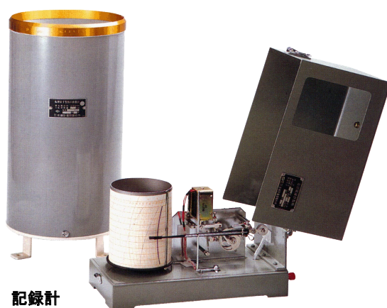
転倒ます型 雨量センサ
