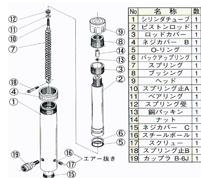
分離式油圧ジャッキ分解図
