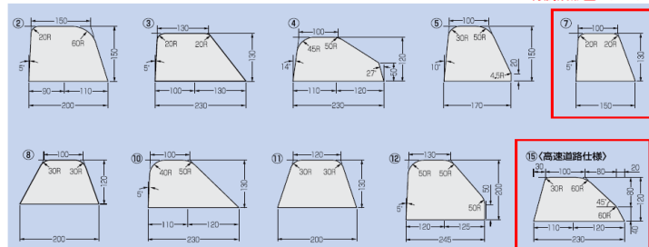
付属成形型・No.7・No.15
