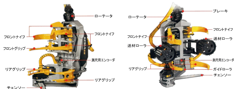
ストロークハーベスタ
