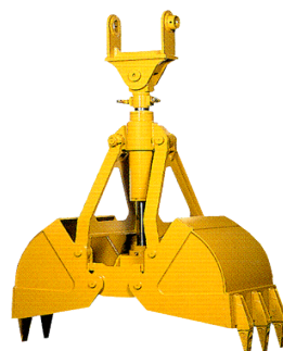
クラムシェルバケット (テレスコプ機械専用) 103216:CSB70-
