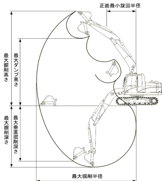
掘削作業範囲図
