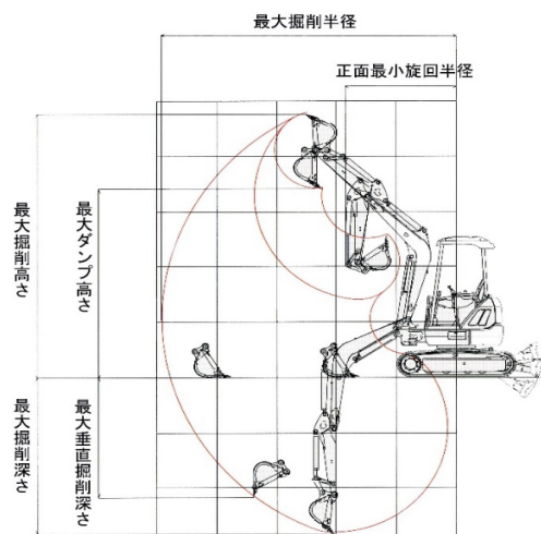
掘削作業範囲図
