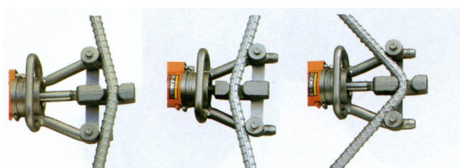
引き修正 押し修正 アンカー曲げ(D32 90°)
