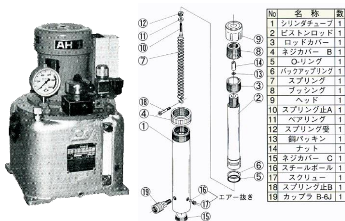
分離式油圧ジャッキ分解図
