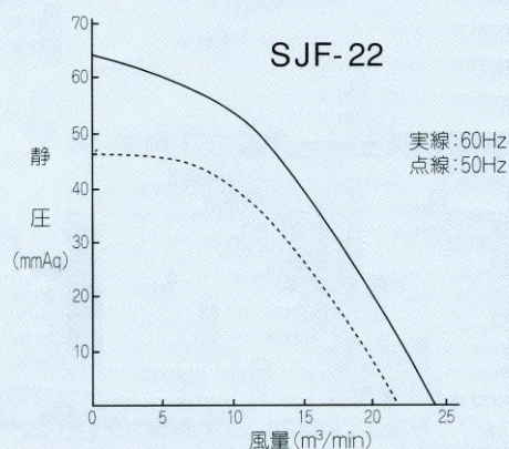
静圧-風量曲線
